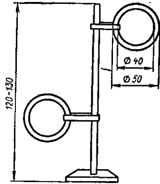
Рис. 58. Стойка для метания в цель
